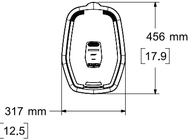
底部視圖
