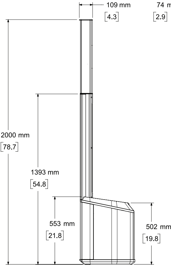
側面視圖
